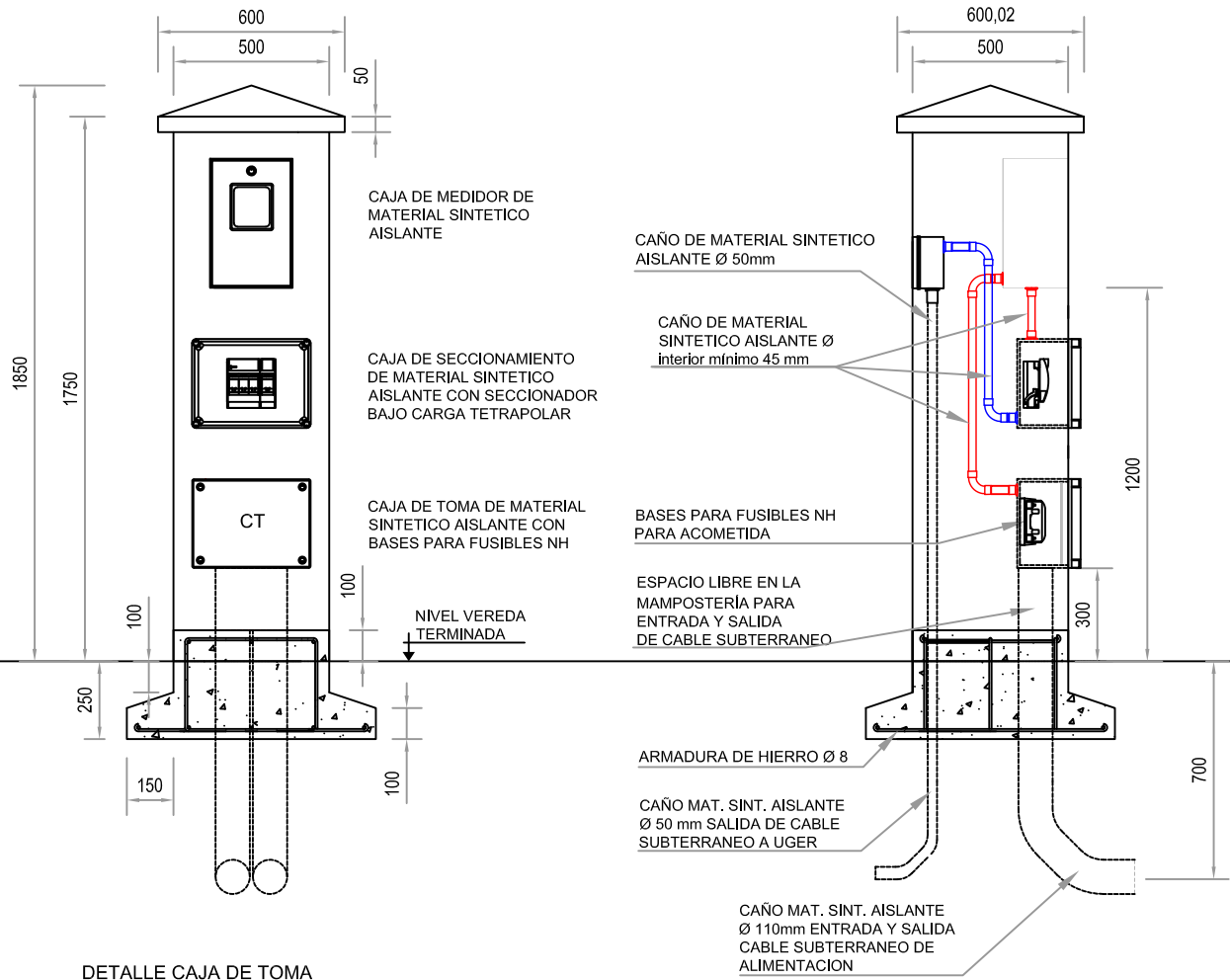
DETALLE CAJA DE TOMA
