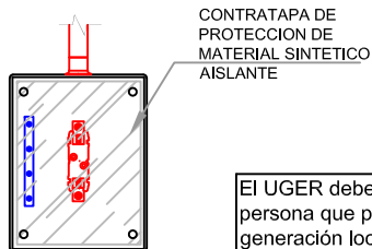
DETALLE CAJA DE TOMA PARA ACOMETIDA SIMPLE
